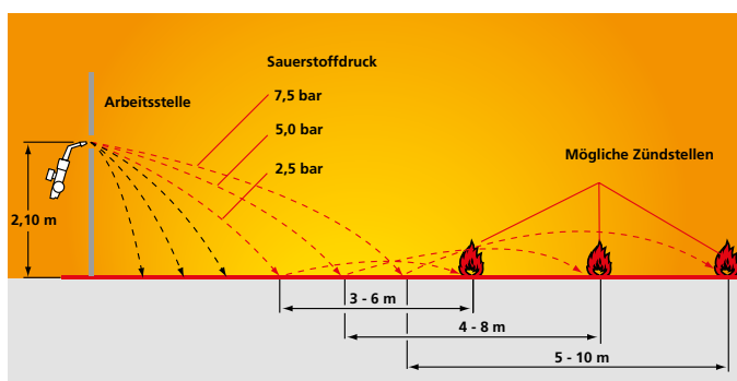
Spritzweite von Schweißperlen - horizontale Reichweite
